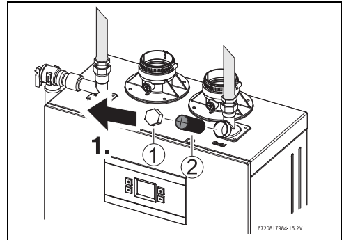
Fig. 29 Filtre à eau
