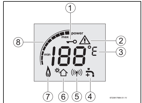
Fig. 41 Description affichage LCD
