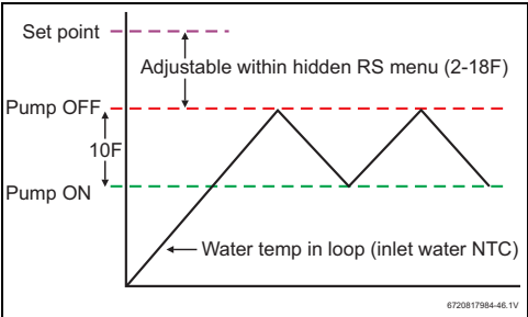
Fig. 31 Intervalles d'activation et désactivation de la pompe
