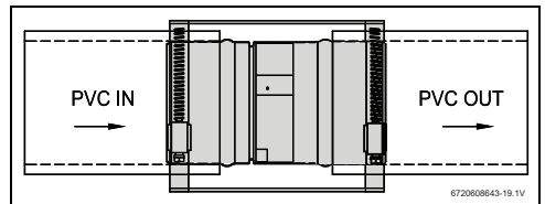
Fig. 22 Réducteur de refoulement (9301BFP) installé
