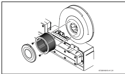
Fig. 54 Retirer/installer le filtre à air
