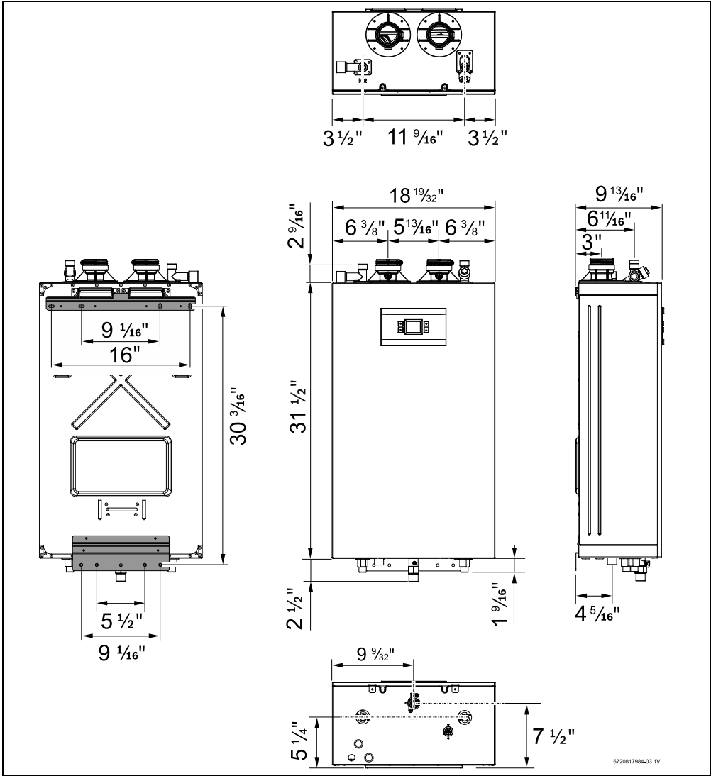
Fig. 5 Dimensions
