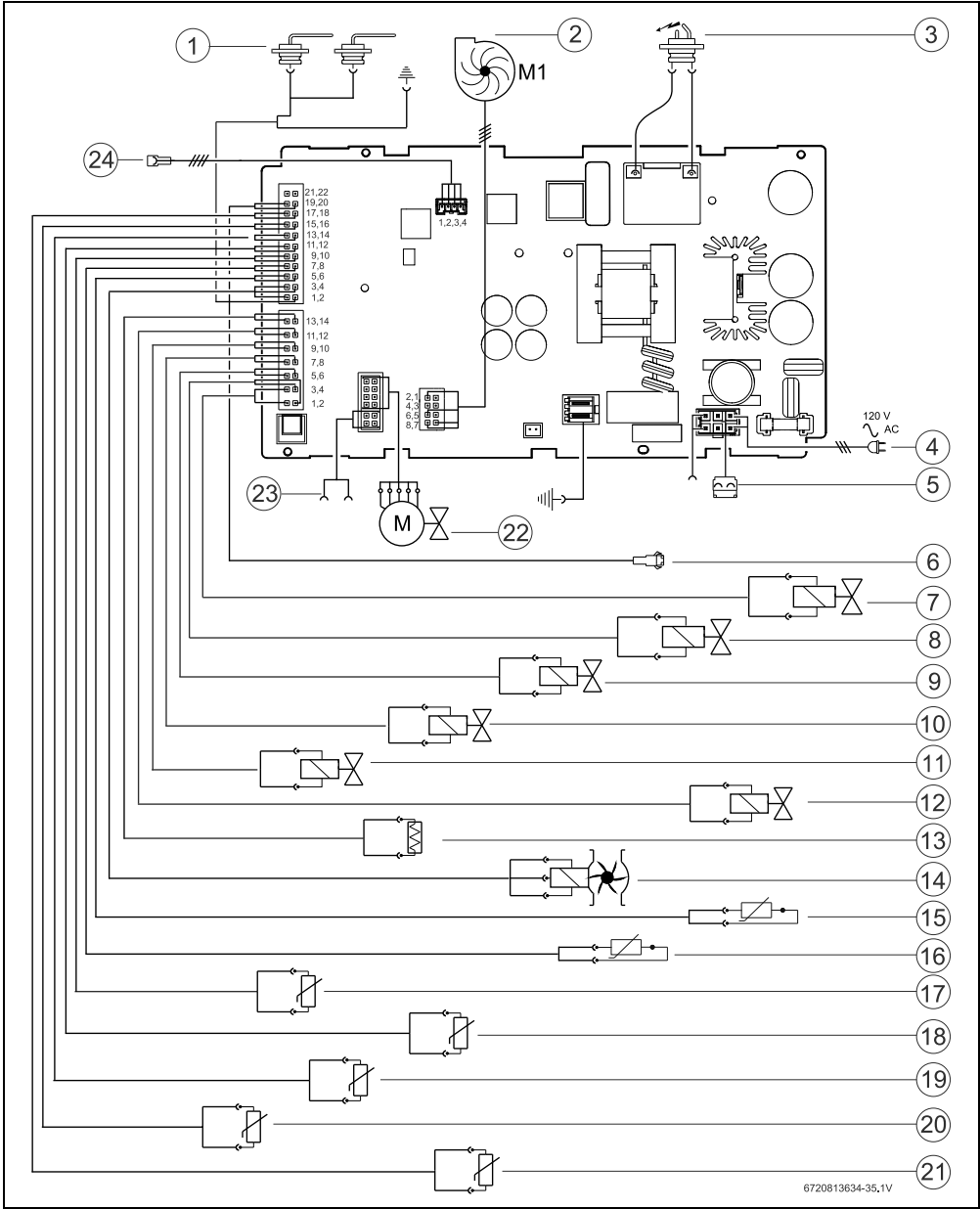
Fig. 62 Schéma électrique
