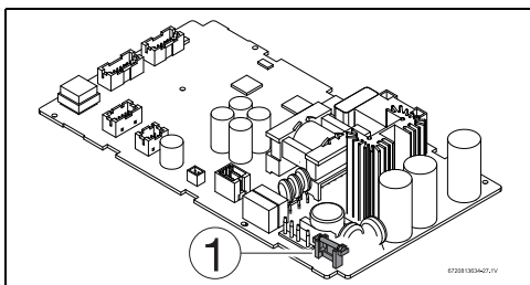
Fig. 39 Position du fusible
