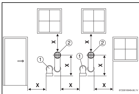
Fig. 17 Position du tuyau d'évent et d'air de combustion d'un système de combustion étanche
