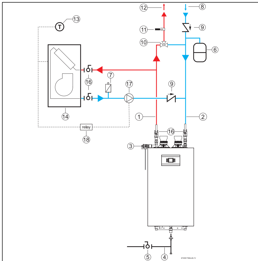
Fig. 34 Système d'air hydraulique avec chauffe-eau
