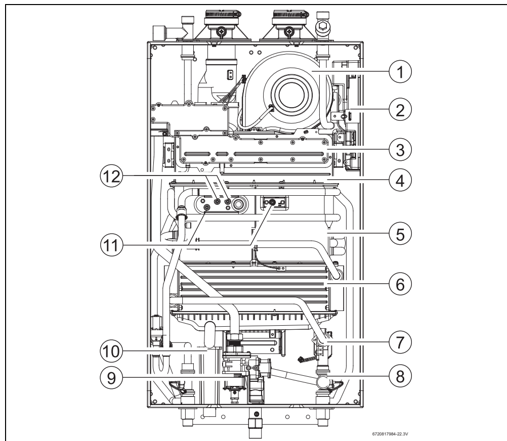
Fig. 66 Composants
