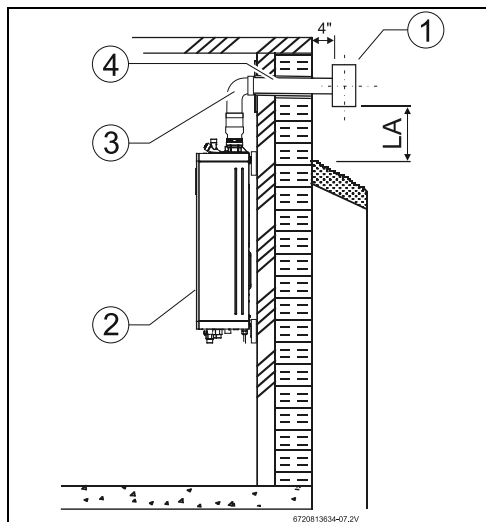
Fig. 15 Installation de ventilation horizontale (tuyau d'air de combustion non illustré)
