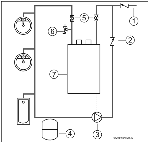
Fig. 30 Application de recirculation avec ligne retour dédiée
