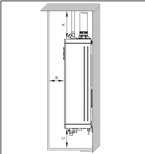
Fig. 6 Vue latérale
