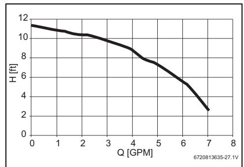
Fig. 32 Courbe hydraulique
