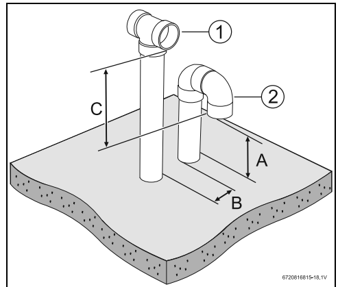
Fig. 13 Système de ventilation verticale
