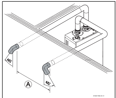
Fig. 14 Système de ventilation horizontale (tuyau double)
