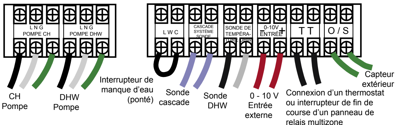
Branchements électriques
