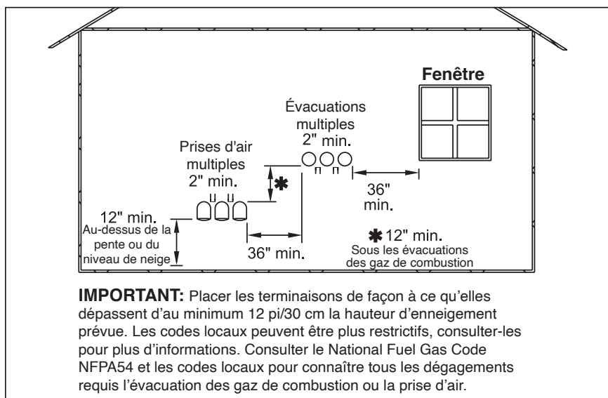
Figure 5. – Plusieurs terminaisons murales latérales, prise d'air et évacuation
