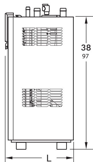
VUE LATÉRALE
