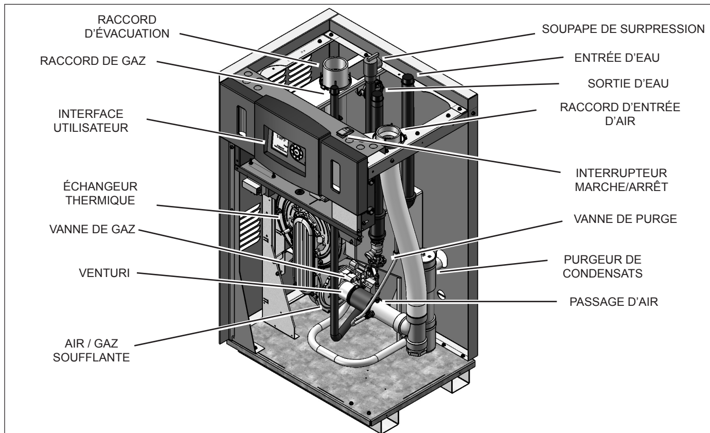
Figure 1. Emplacement des composants, puissances 80–210
