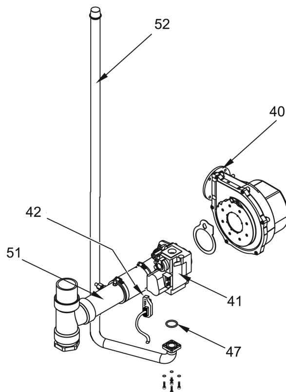
Figure 41. – Composants du circuit de gaz, puissances 80–285
