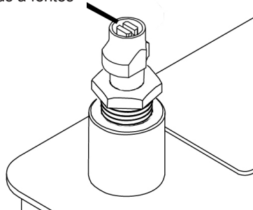
Figure 36. Purge d'air
