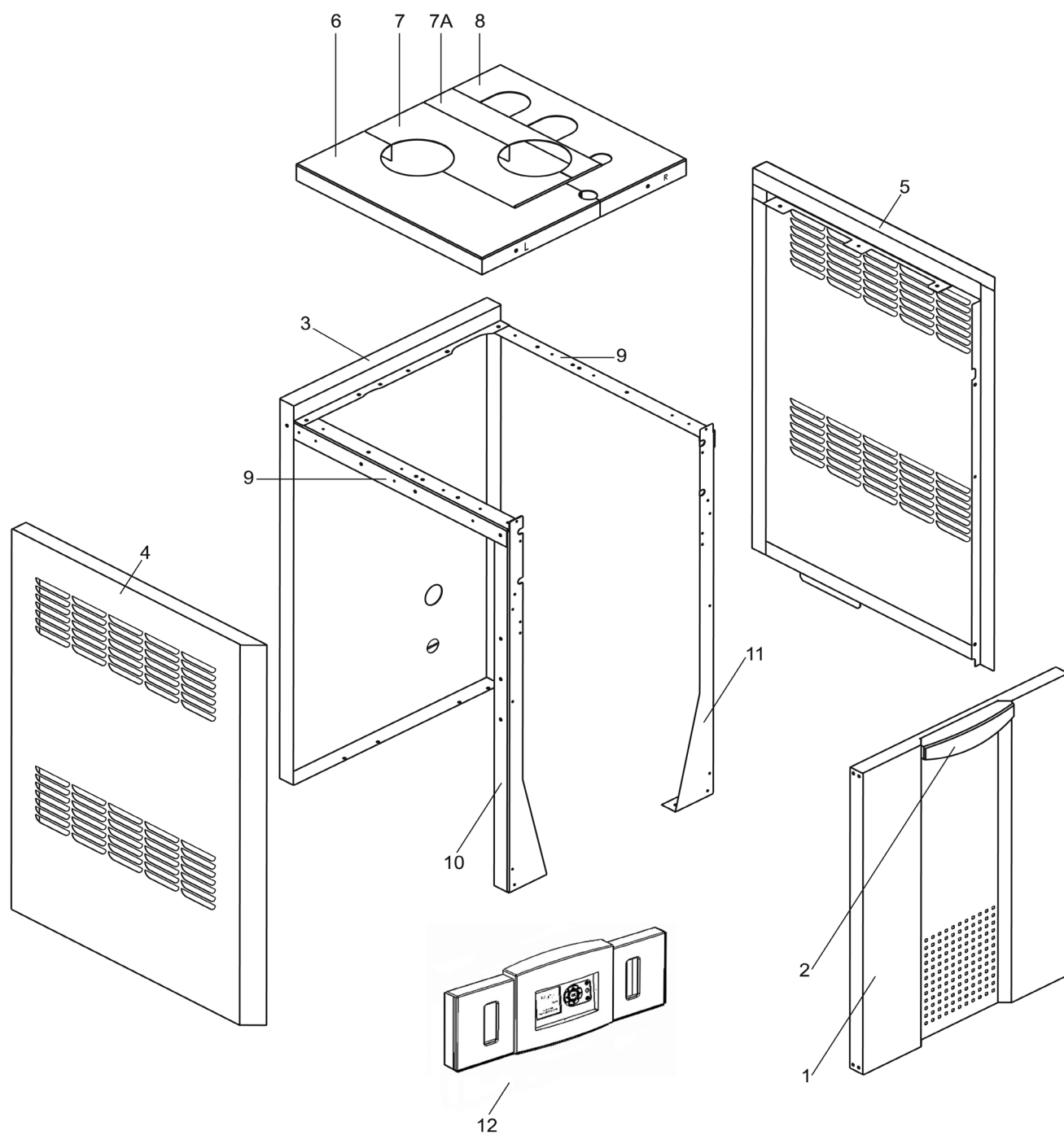
Figure 40. – Composants de l'enveloppe
