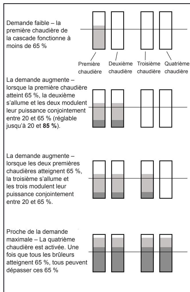
Figure 34. Cascade (Lead Lag), 4 chaudières ou plus.
