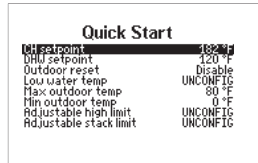
Figure 27. – Menu Démarrage rapide (Quick Start)
