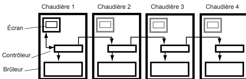
Figure 32. Cascade « Lead Lag » dans un système à quatre chaudières. Remarque: pour les chaudières 2 à 4, l'écran tactile affiche uniquement les informations relatives à chaque chaudière concernée.
