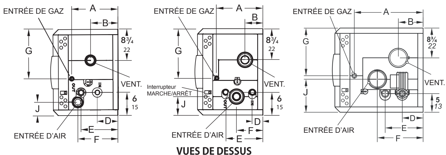
MODÈLES 080 et 105
